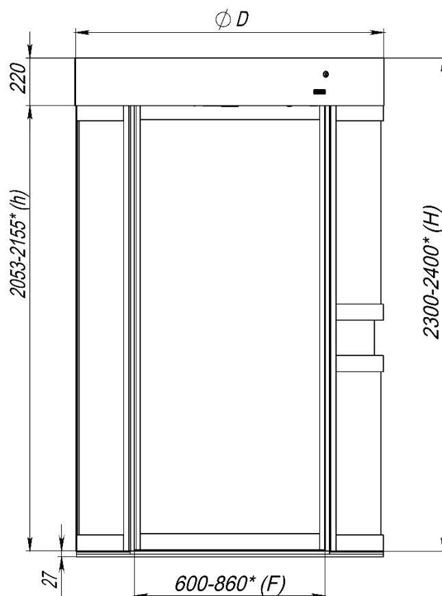
Рисунок 1. Габаритные размеры шлюзовой кабины ГАРТЕК ЦАН – ХХ00-А
